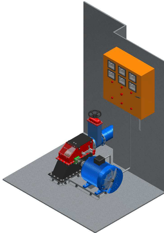
Figura 3. Vista general del prototipo ensamblado de la turbina Michell-Banki
