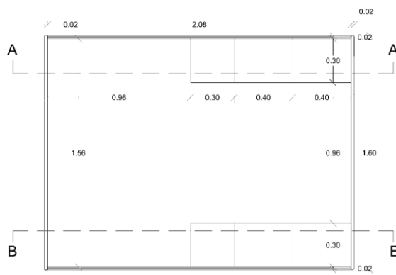
Planta
