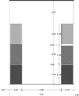
Alzado
